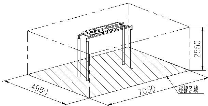
器材最小空间示意图
